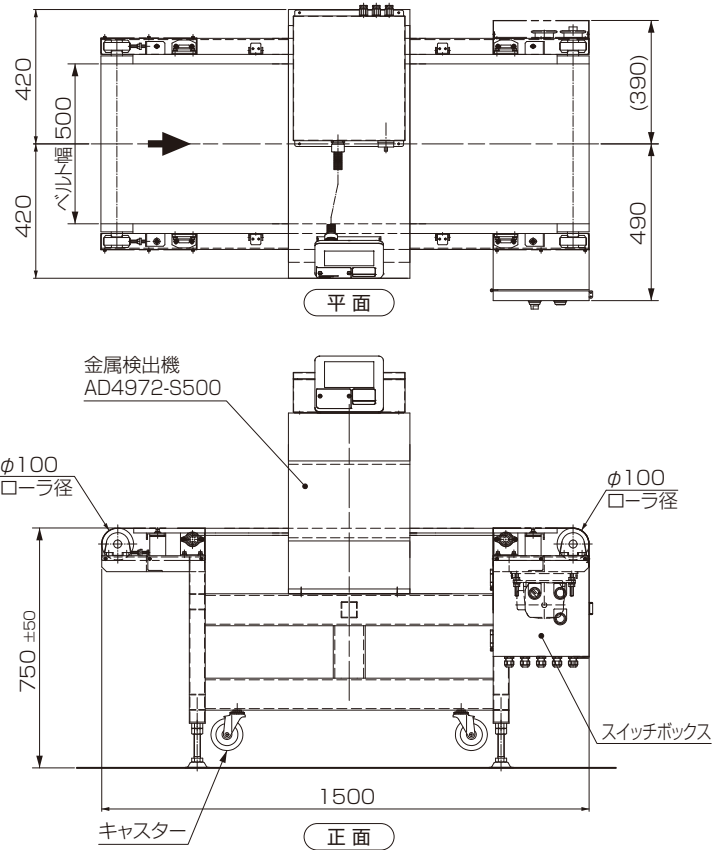
AD4972-S500 外観図
