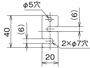
ケーブルクランプ詳細図
