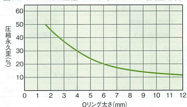
図1-2 25%圧縮 A305 (120°C 70時間空気中)
