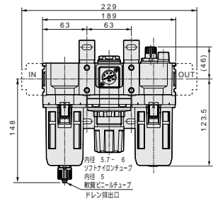
W3000外形寸法
