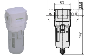
R3000外形寸法
