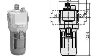
L3000外形寸法
