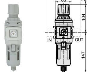
W3000外形寸法
