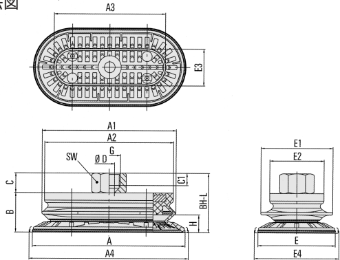
寸法図
