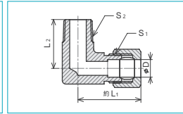
RMLおねじエルボコネクタ
