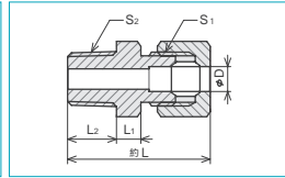
RMCおねじコネクタ
