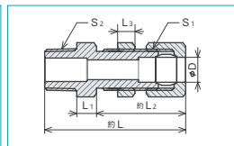
RMB隔壁型おねじコネクタ
