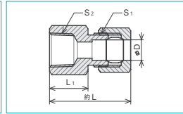
RFCめねじコネクタ
