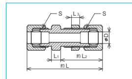
RUB隔壁型ユニオン
