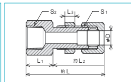
RFB隔壁型めねじコネクタ
