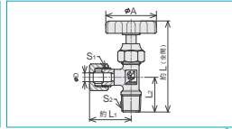
VRZ弁棒ロックタイプ
