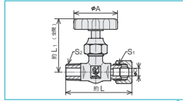
VRY弁棒ロックタイプ
