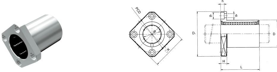
LMK/LMK-M形
