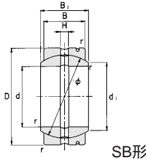
SB形
