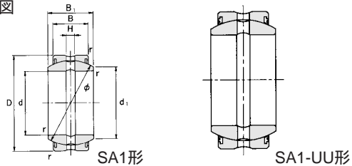
SA1形
