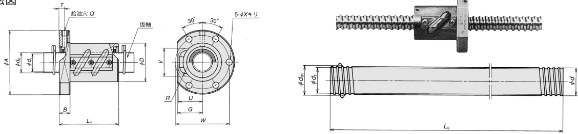
寸法図
