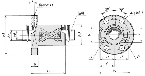
RNFTL寸法図
