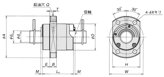
RNFCL寸法図
