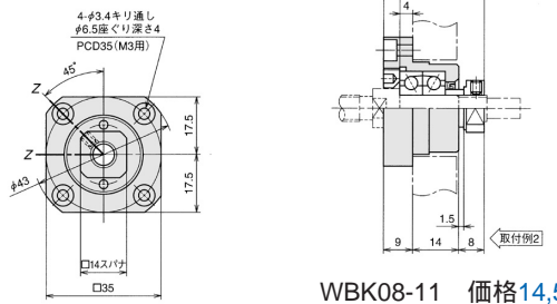
WBK08-11 価格14,500
