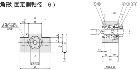
WBK06-01A 価格13,400
