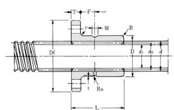
TMF-OH形
