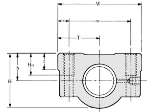
TMH形
