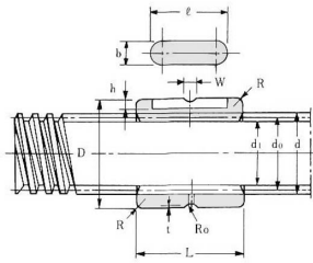
TMS-OH形
