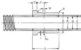
TMK-OH形
