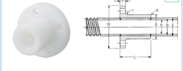
TMF-P形プラスチックナット寸法価格 材質:ポリアセタール
