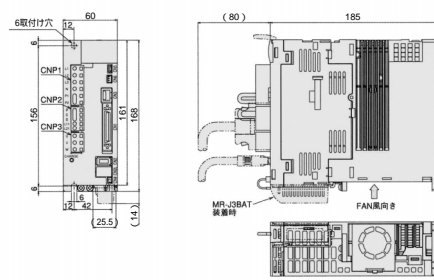
MR-J3-70A, 100A
