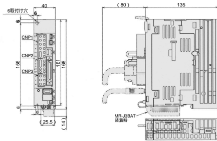
MR-J3-10A, 20A
