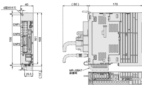
MR-J3-40A, 60A
