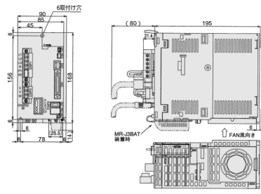
MR-J3-200A, 350A
