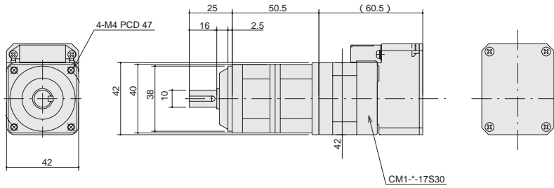
CMG-17S-03 05/09 S型寸法図
