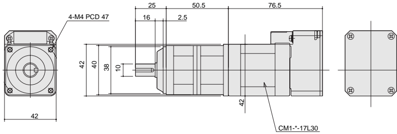
CMG-17L-03 05/09 S型寸法図
