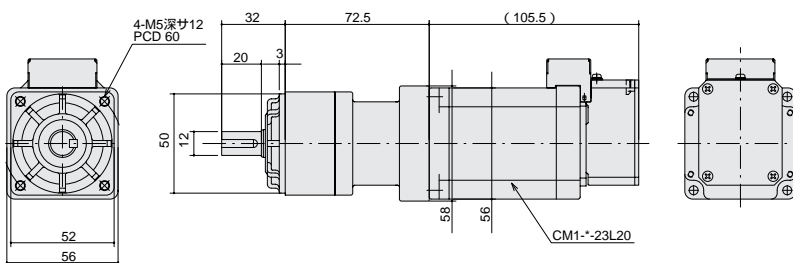
CMG-23L-03 05/09 S型寸法図
