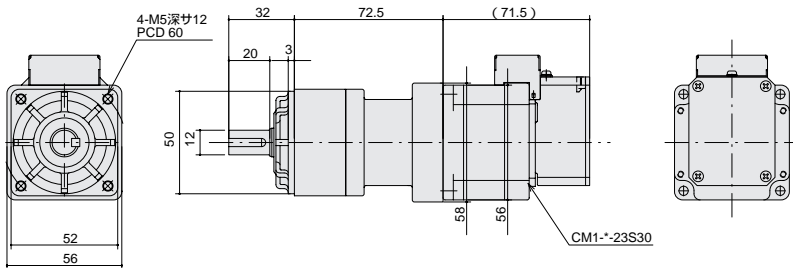
CMG-23S-03 05/09 S型寸法図
