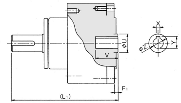
SH型(入力軸差し込みキー止めタイプ)
