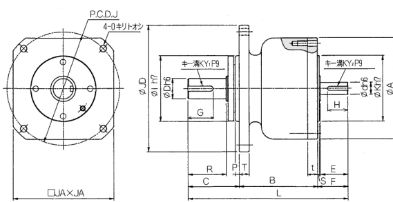
SS型 入力軸シャフトタイプ)
