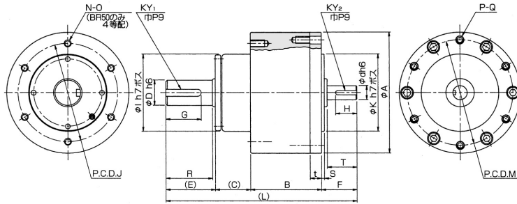
SS型(入力軸シャフトタイプ)
