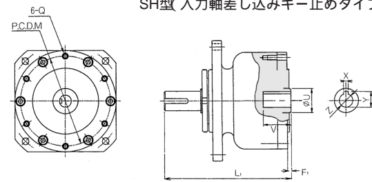
SH型 入力軸差し込みキー止めタイプ)
