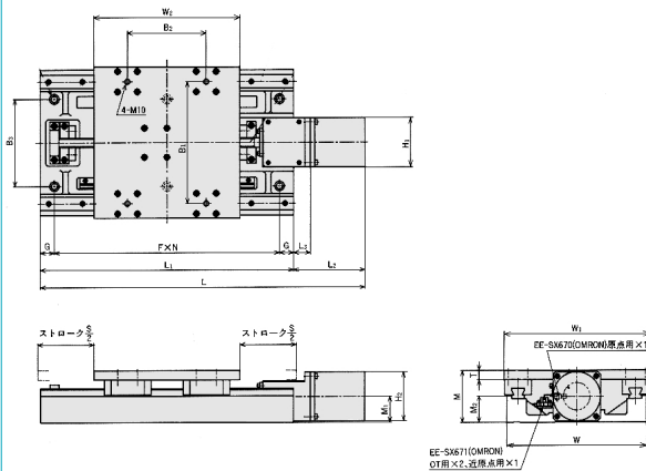
寸法図(A20 ~ A50)
