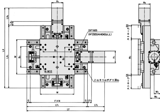
寸法図(AX2020 ~ AX5050)
