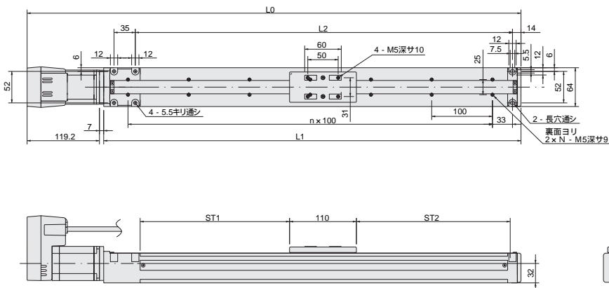
RL2-60T20型寸法図
