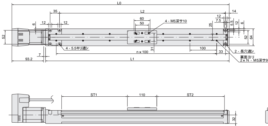
RL2-60T10型寸法図
