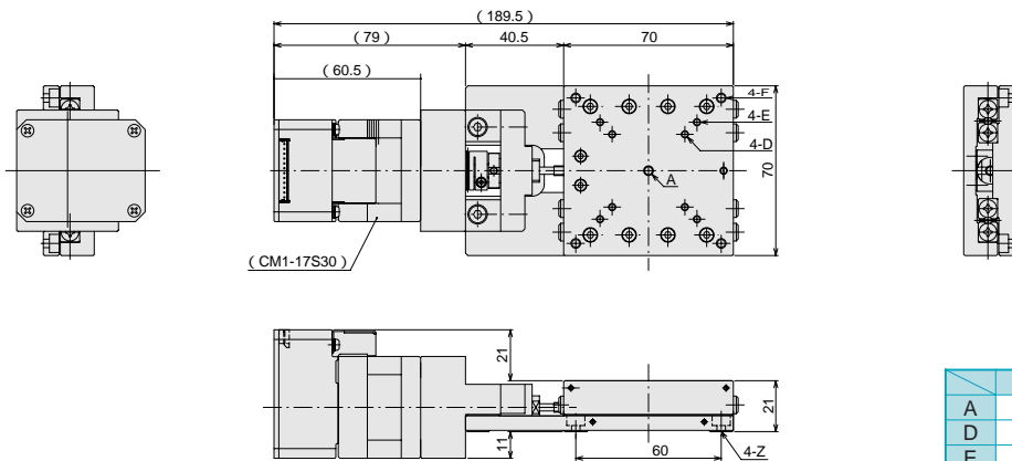
CR-7070-10型寸法図
