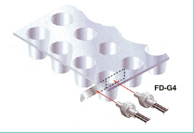
シロップ容器の位置決め (FD-G4)
