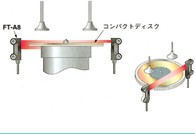
コンパクトディスクの2枚重なり検出 (FT-A8)
