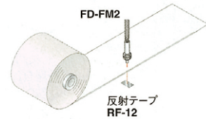
半透明シートの有無検出
