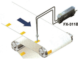
レジマークの有無検出
