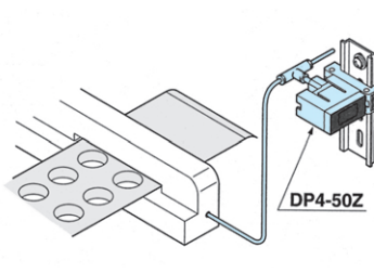
真空成形の真空度確認
