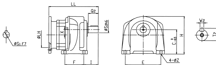
寸法図
