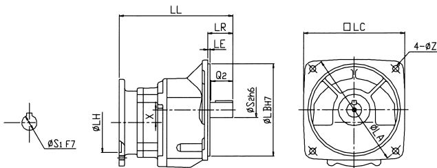
寸法図
