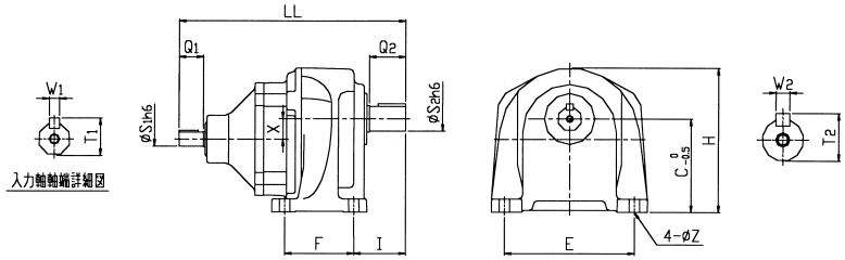
寸法図
