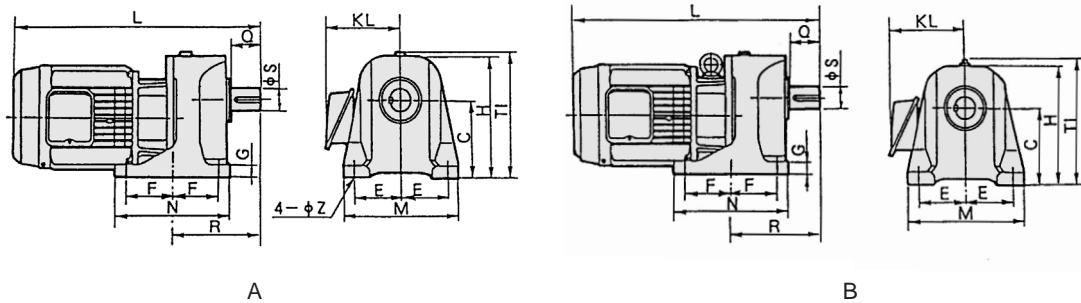
寸法図
