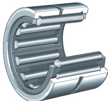
RNA49-2RSR形
