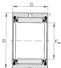
RNA49-2RSR形
