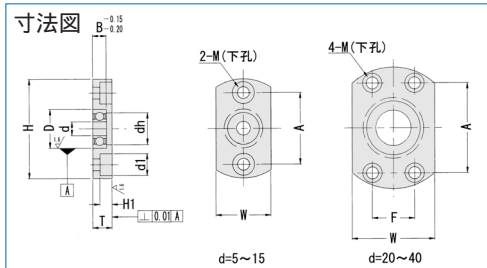
BES型 (SUS)
