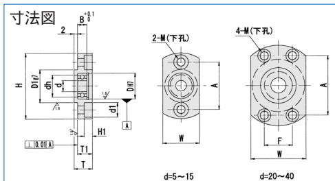
BEIS型 (SUS)
