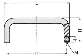
PHPF形パネルハンドル ステンレスSUS304、パフ研磨
