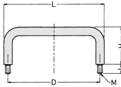
PHP形パネルハンドル ステンレスSUS304、パフ研磨
