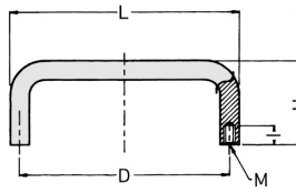
PBHF形パネルブラックハンドル 黄銅C3604特殊コーティング
