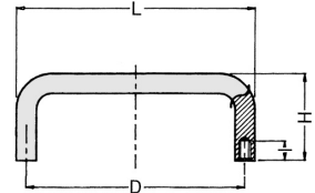
RHPF形ラウンドハンドル ステンレスSUS303、パフ研磨
