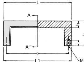
SHPF形スクウェアハンドル 亜鉛ダイキャストクロムメッキ
