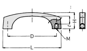
AHP形・AHPF形アーチハンドル 亜鉛ダイキャストクロムメッキ
