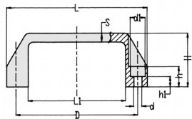
AGS形アーチグリップ 艶消し黒色ナイロン樹脂
