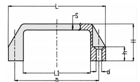
AGS-N形アーチグリップ 艶消し黒色ナイロン樹脂
