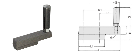
ABH-N型 アルミニウムバランスハンドル ●ボディ: アルミ
