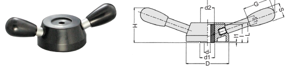
TA型 ツーアームハンドル ●ボス: ナイロン樹脂、インサート: SUM22L
