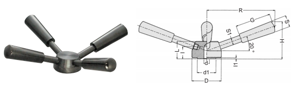
FA型 フォーアームハンドル ●ボス: 鋼材S45C
