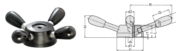
FA型 フォーアームハンドル ●ボス: ナイロン樹脂、インサート: SUM22L
