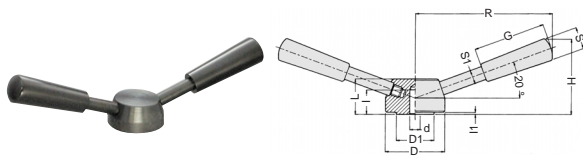
TA型 ツーアームハンドル ●ボス: 鋼材S45C
