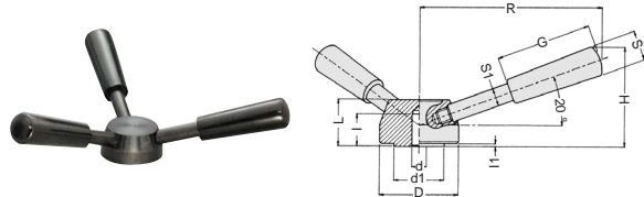
TRA型 スリーアームハンドル ●ボス: 鋼材S45C
