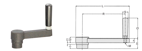
ACH-N型 アルミニウムクランクハンドル ●ボディ: アルミ
