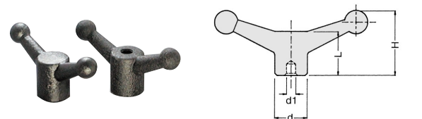
SH型 スピードハンドル ●ボディ: タグタイル 鋳鉄FCD45
