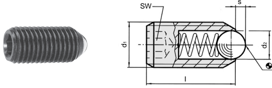
EH2203形標準圧 (ボール付 六角穴付)
