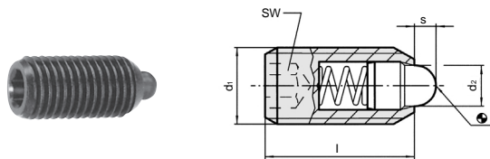
EH2203形標準圧 (スラストピン付 六角穴付)
