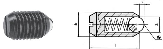
EH2205形標準圧 (ボール付, スロット付)
