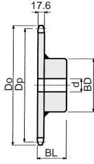
B型(溶接仕様)
