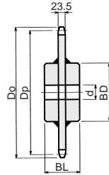
C型(両ボス)
