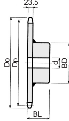
B型(溶接仕様)
