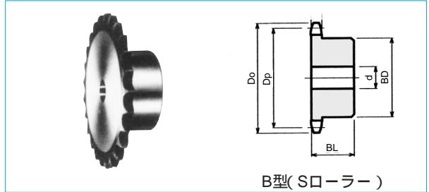
B型( Sローラー )
