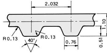
寸法図
