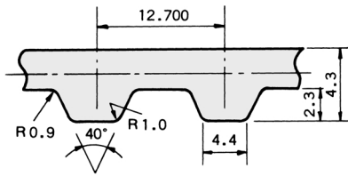
H形標準歯形形状
