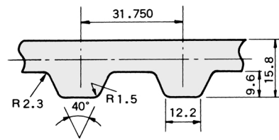
XXH形標準歯形形状
