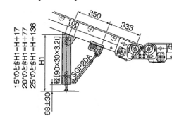
EF形 傾斜)
