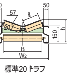
標準20トラフ
