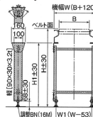
EF形 水平)
