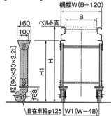
EC形 水平)
