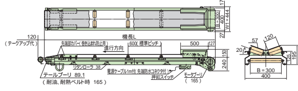
SBT形標準図
