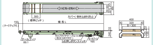
SBF形標準図
