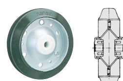
ゴム軸受、ポリアセタール軸受
