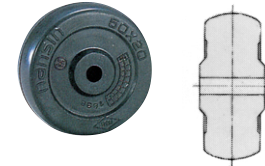
一体ゴム車輪
