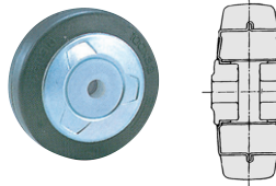
ポリアセタール軸受、鋼板ホイール
