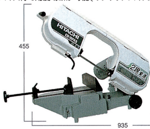
帯のご刃寸法: 周長1,840×幅12.5×厚さ0.65mm パイプ外径: 180mm CB18FA3 価格 275,000
