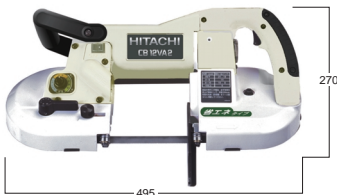
帯のご寸法: 周長1,130×幅12.5×厚さ0.5mm パイプ外径: 120mm CB12VA2 価格 78,700 (保護カバー付)
