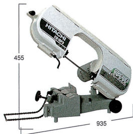
帯のご刃寸法: 周長1,840×幅12.5×厚さ0.65mm パイプ外径: 180mm CB18F3 価格 273,300
