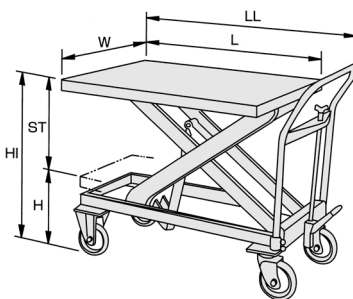
寸法図
