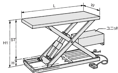
寸法図
