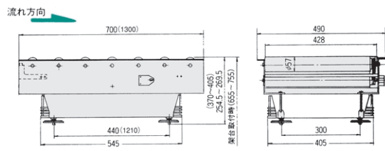
AD-4942A-30K、35K寸法図( )内寸法35Kタイプ
