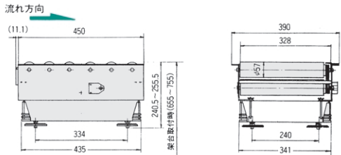
AD-4942A-15K寸法図
