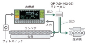
選別機を連動させる例
